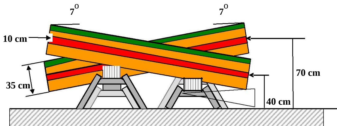
Slika 11. Postavljanje trupaca (kuta) i promjeri
